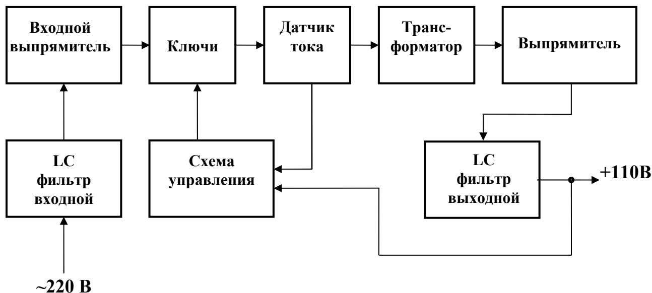
Рис.1. Структурная схема ИПС-300.
